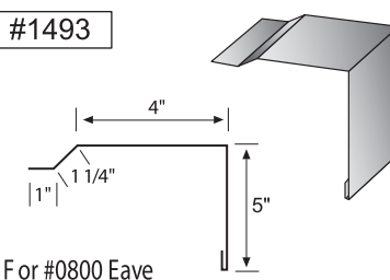
CF &amp; AP Rake
