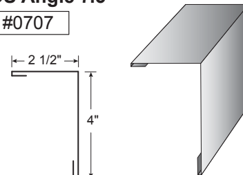
OS Angle 7.5"
