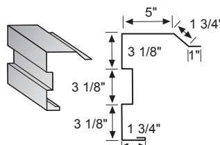
CP High Side Rake
