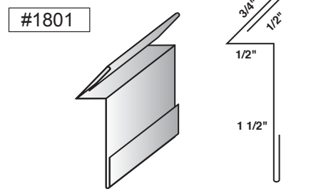
SS MLK Rake Slide
