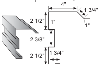
CP Rake Trim
