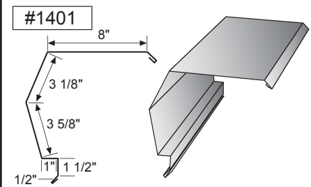
SS Rake
