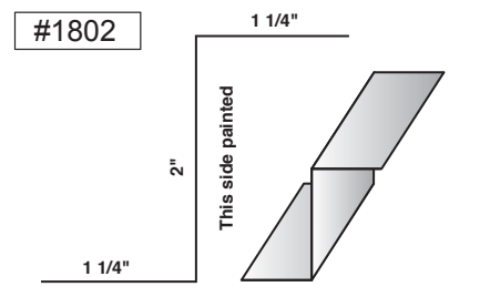
SS Rake Zee
