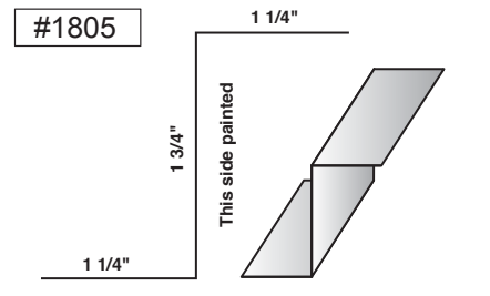
SS MSL Rake Zee
