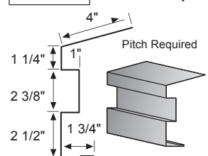
CP Low Side Eave
