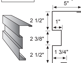
CP High Side Rake
