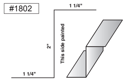
SS Rake Zee
