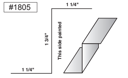
SS MSL Rake Zee
