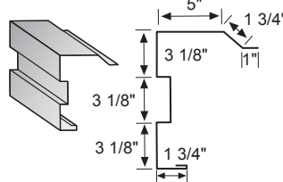
CP High Side Rake
