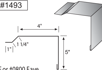
CF &amp; AP Rake
