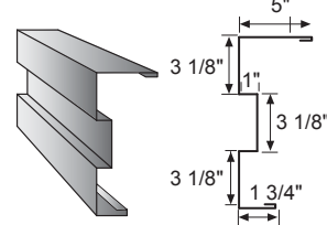
CP Low Side Eave
